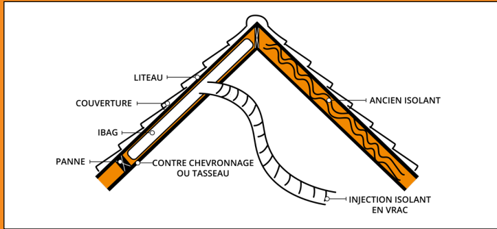
Isolation des combles aménagés depuis l'intérieur avec l'Ibag
