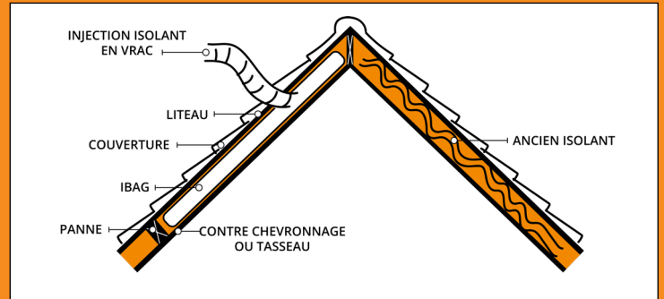
Isolation des combles aménagés depuis l'extérieur avec l'Ibag
